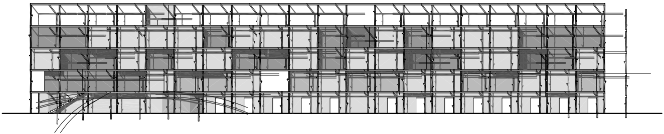
ANSICHT-SÜD 1:250, FENSTERTEILUNG 1:100 ALTMANNSDÖRFER ANGER PLANUNGSSTUDIE I
