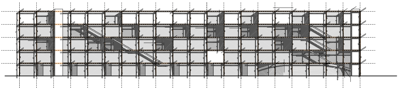
ANSICHT-NORD, SYSTEMSCHNITTE 1:250 ALTMANNSDÖRFER ANGER PLANUNGSSTUDIE I
